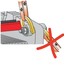
Abbildung 9: Hebevorrichtung für AQ20S. Die vier inneren Ösen beim Anheben des Wärmeübertragers verwenden. Die Transportbefestigungspunkte dürfen NICHT verwendet werden! Befestigungsvorrichtung wird benötigt.
