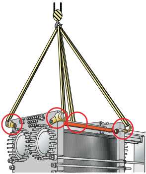
Abbildung 8: Hebevorrichtung für AQ20. Befestigungsvorrichtung wird benötigt.
