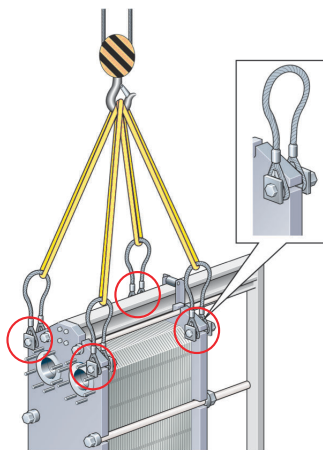
Abbildung 6: Hebevorrichtung für AQ14 und AQ14S. Befestigungsvorrichtung wird benötigt.
