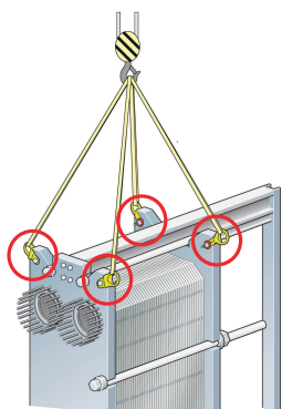
Abbildung 6: Hebevorrichtung für T45, TL35 und WideGap 350. Befestigungsvorrichtung wird nicht benötigt.
