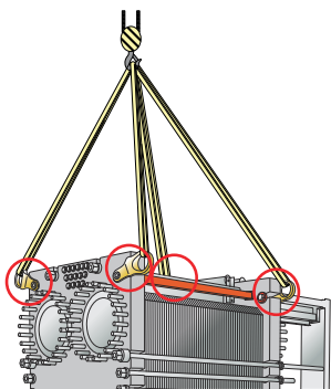
Abbildung 7: Hebevorrichtung für T50. Befestigungsvorrichtung wird benötigt.
