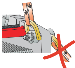
Abbildung 8: Hebevorrichtung für TS50. Die vier inneren Ösen beim Anheben des Wärmeübertragers verwenden. Die Transportbefestigungspunkte dürfen NICHT verwendet werden! Befestigungsvorrichtung wird benötigt.
